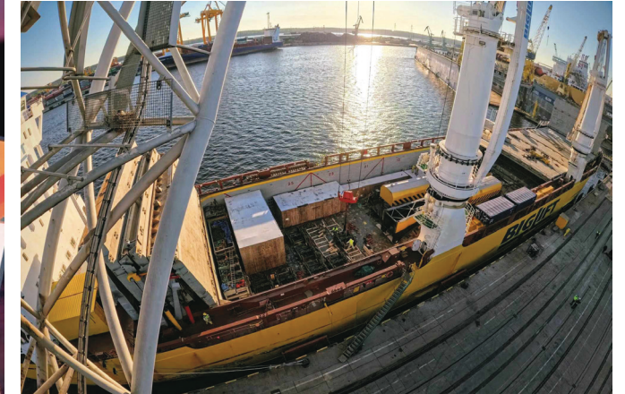
Der komplizierte Transport beinhaltete zahlreiche verschiedene Transportmittel und die komplette Zerlegung des Synchronkondensators.
